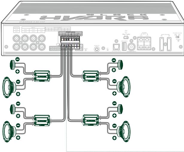
Пример 1. Speakers outputs: 2x-полосный фронт + 2x-полосный тыл.
