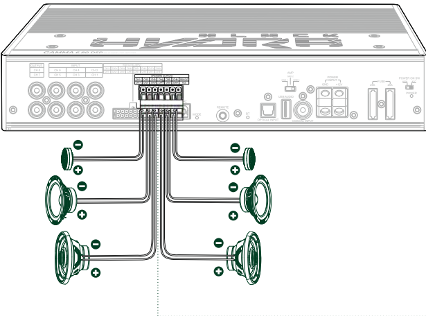
Пример 2. Speakers outputs: 2x-полосный фронт + широкополосный тыл.
