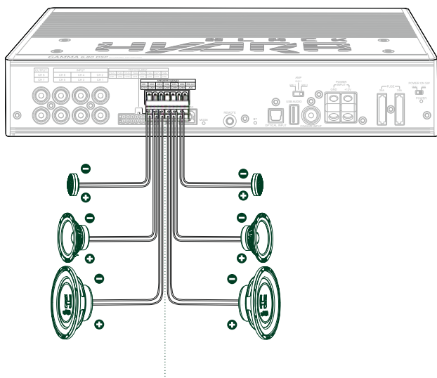
Пример 3. Speakers outputs: 2х-полосный фронт + два сабвуфера.
